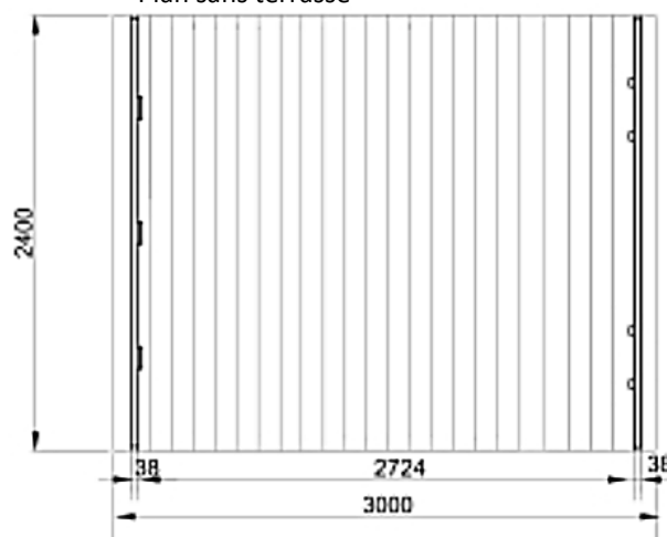
Plan sans terrasse
