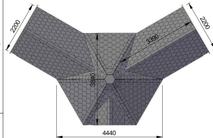
PLAN DE COUPE 3D
